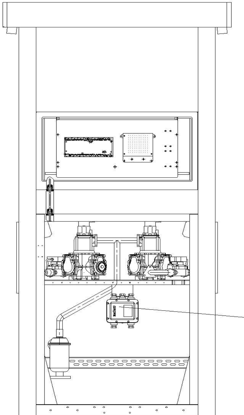
1 - клеммная коробка
